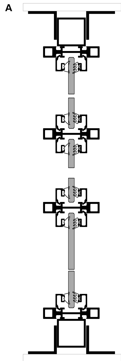
Secțiune verticală
